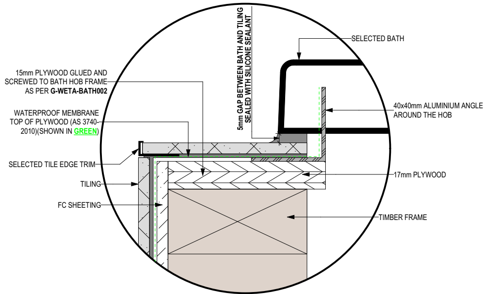
DETAIL 01 SCALE: 1:2
