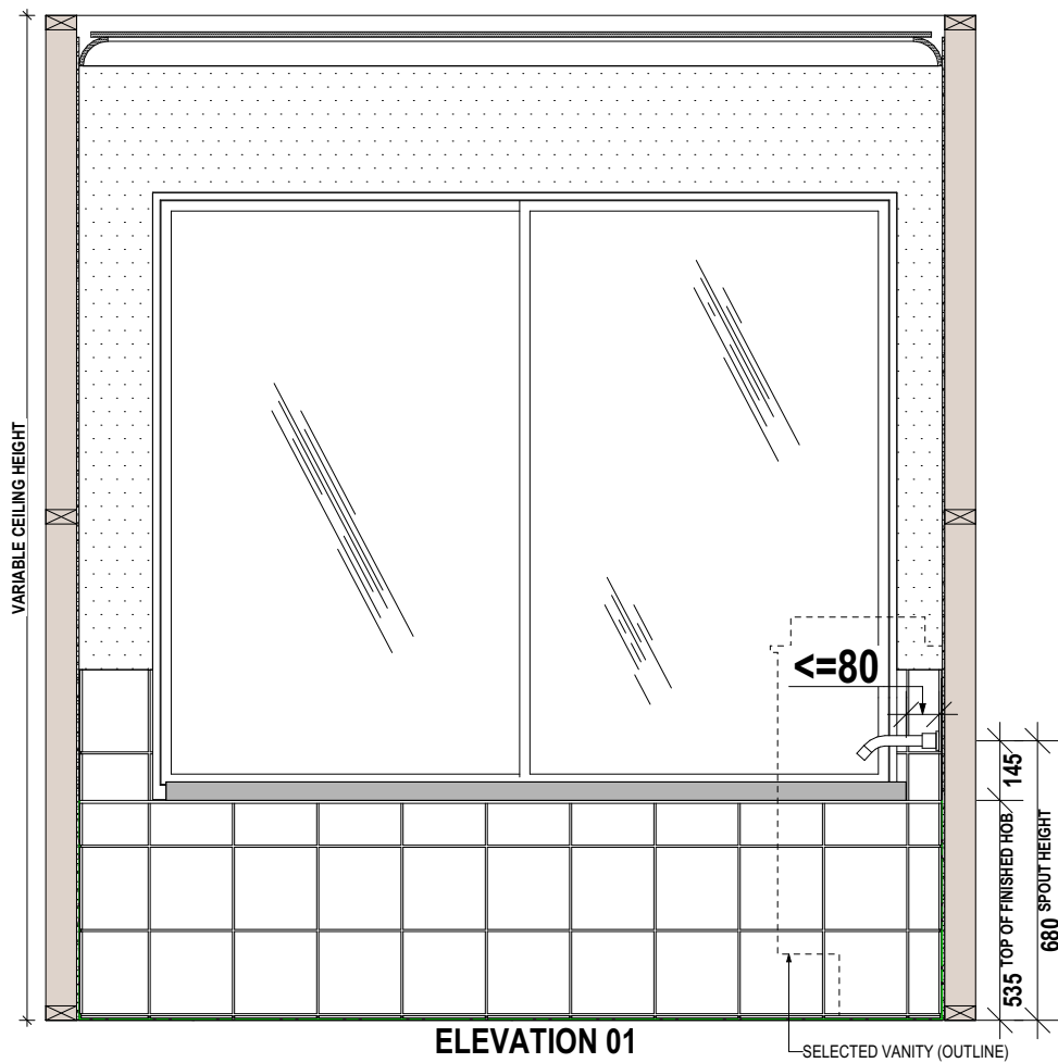
SECTION 01 SCALE: 1:10
